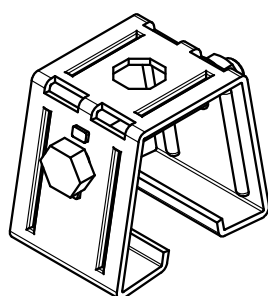
HY-T1斜視図
